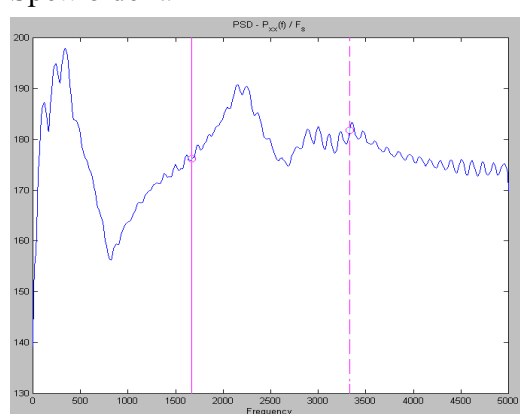
Spettro della 'i'
