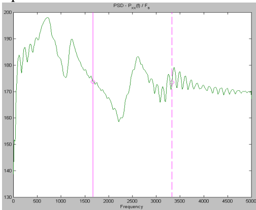
Spettro della 'a'
