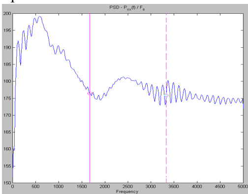
Spettro della 'O'
