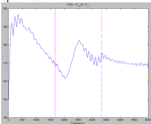
Spettro della 'u'
