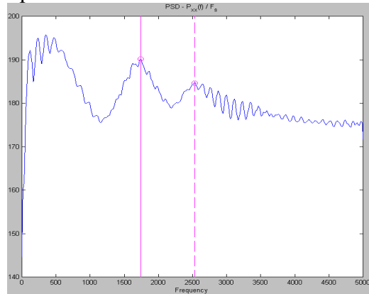
Spettro della 'e'
