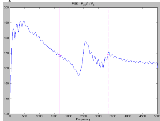
Spettro della 'o'
