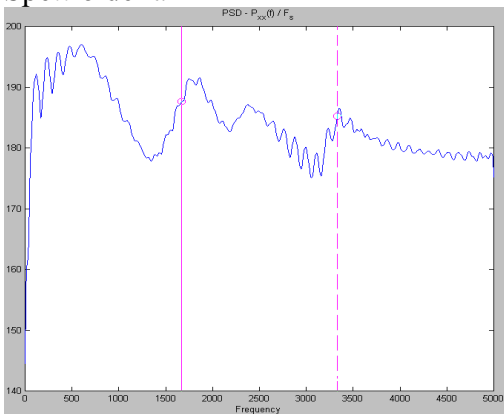
Spettro della 'E'
